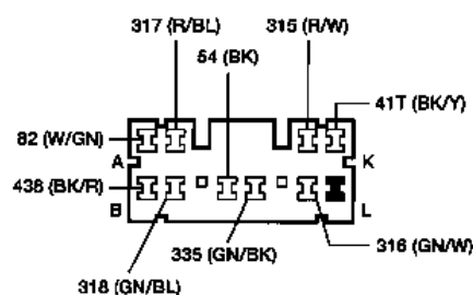
LEFT POWER DOOR LOCK SWITCH
